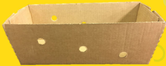
MB1PA01-44 - 5lb Box Glued (1155/skid)
